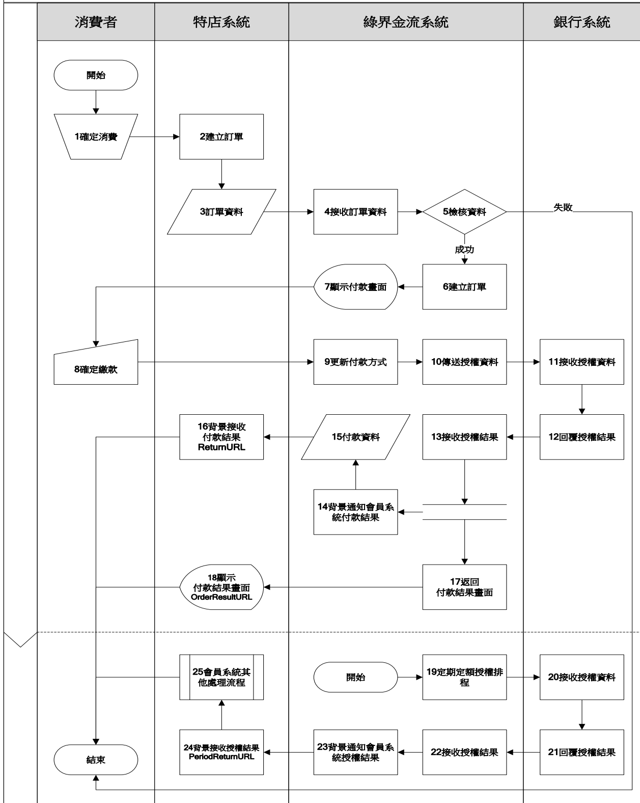
[圖 2-3]信用卡定期定額系統介接循序圖
